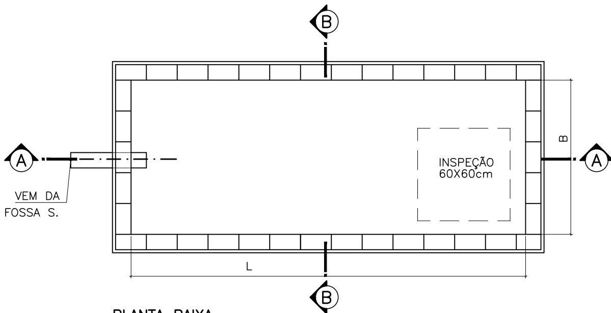
PLANTA BAIXA
