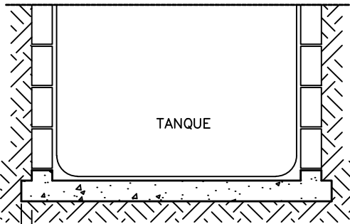
JUNÇÃO LAJE DE FUNDO/PAREDES LATERAIS
